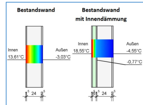
Innendämmung
